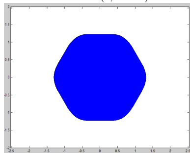
FIG. 4.4. A(9, e^{2\pi i/3}) .
